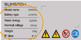
Battery Module
