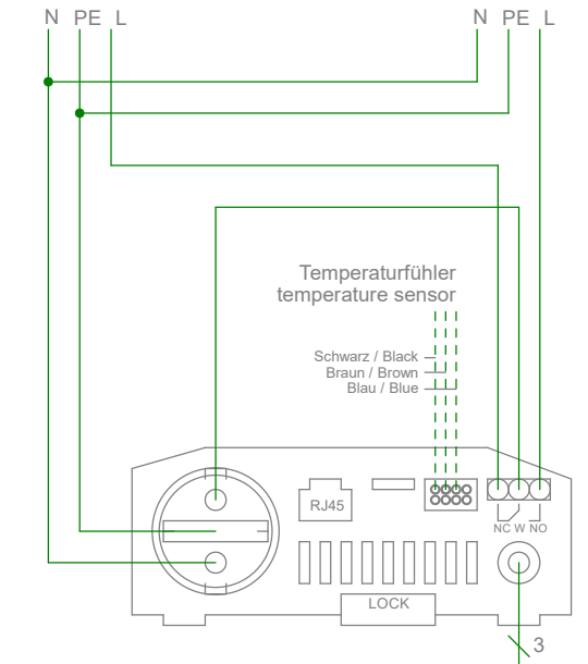
Unterseite / Bottom View
